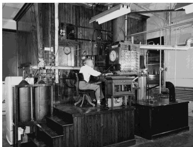
Figura 1. Calorímetro de Armsby (1917)
