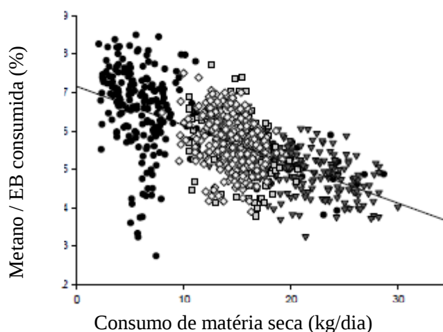
Figura 8. Fonte: Adaptado de Mills et al. (2009). Relação entre consumo de matéria seca e emissão de metano como porcentagem da energia bruta (EB) consumida em bovinos
