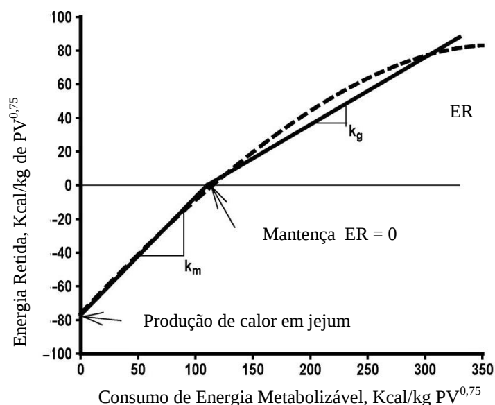
Figura 3. Representação da relação entre energia retida (ER) e consumo de energia metabolizável (EM). A linha tracejada mostra a relação curvilínea entre a ER e EM derivada à partir da relação entre o logaritmo da produção de calor e o consumo de EM (Garrett, 1980); a linha sólida mostra uma aproximação linear (NRC, 1981).
